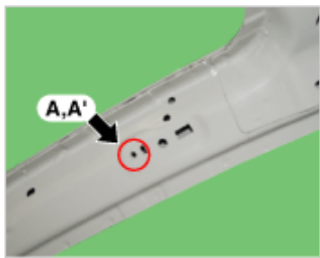
窗帘式空气囊装配孔 (Ø6.6)
